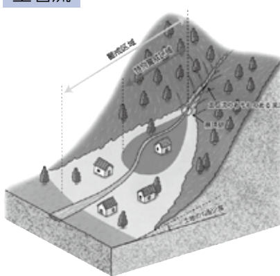
土石流
