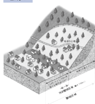
地滑り
