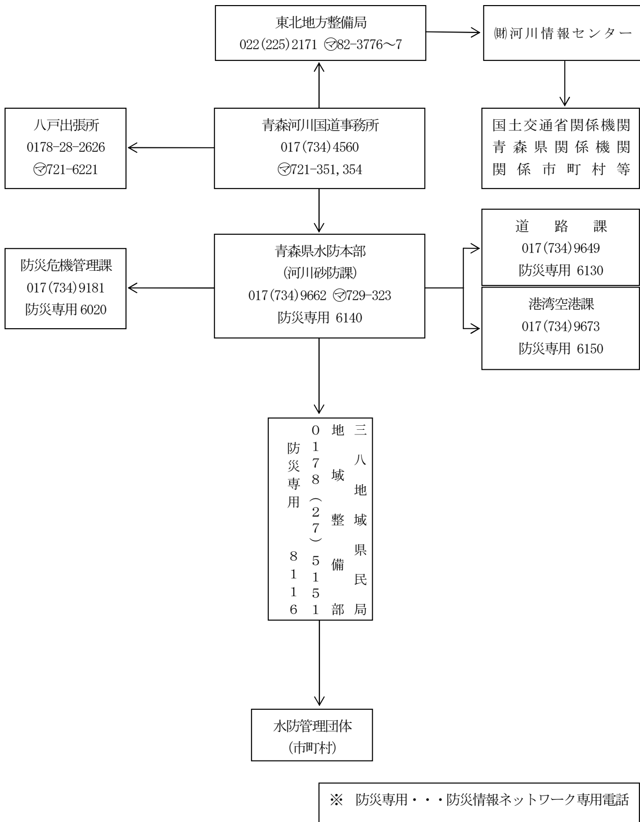
【水防警報伝達系統図（国土交通省）馬淵川水防警報伝達系統図】
