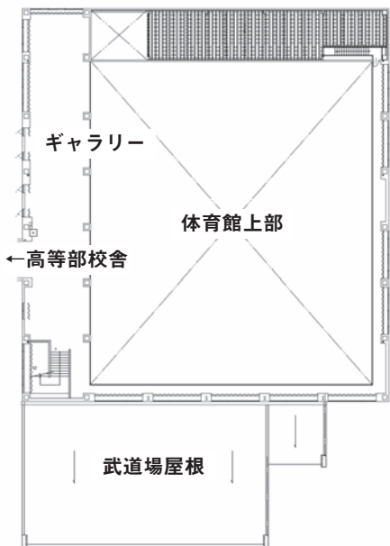
2階平面図
